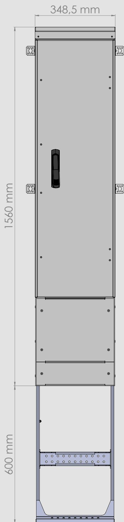
Enkelt
